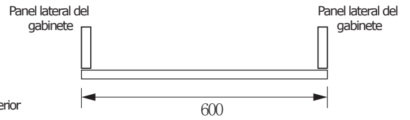
Referencia e indicación del tamaño de la puerta superpuesta completa
