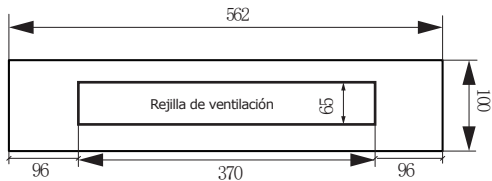
Diagrama esquemático del zócalo
